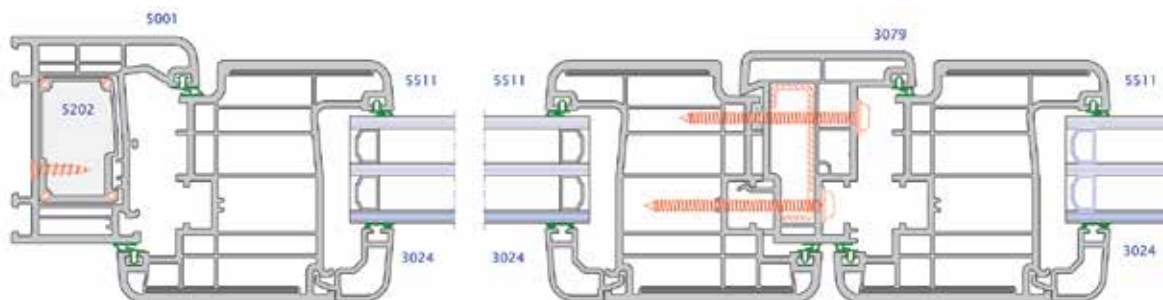
Secção horizontal do sistema OpenMAX Premium
